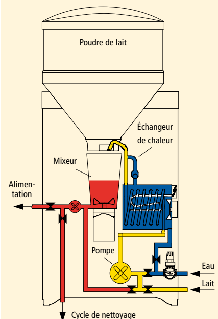
Distributeur d'alimentation combi lait+ poudre pour veaux.
